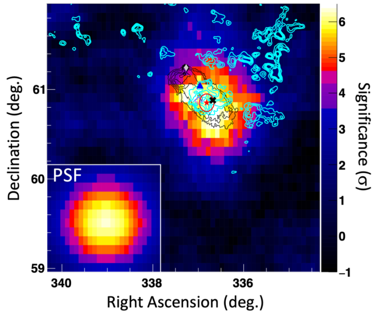
図 3 チベット空気シャワー観測装置で見た超新星残骸 G106.3+2.7 方向の 10TeV 以上のガンマ線イメージ。PSF は装置の角度分解能によるひろがりを示す。黒の等高線は超新星残骸の外殻、水色の等高線は分子雲の分布、灰色のダイヤモンドはパルサーの位置を示す。赤の星印(統計誤差を示す円付き)、黒の✱印、マゼンタの十字および青の三角は、チベット空気シャワー観測装置、Fermi 衛星、VERITAS チェレンコフ望遠鏡および HAWC 実験で観測されたガンマ線放射領域の中心をそれぞれ示す。
