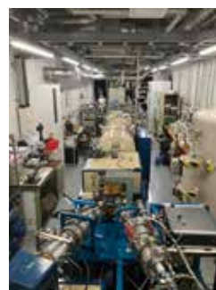
研究室の全景。中央が1MVのタンデム型イオン加速器(手前から奥に向かって加速)。高速イオンビームを用いた元素分析やビーム照射による改質を行うことができます。
